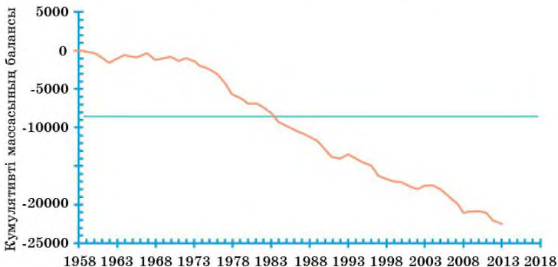
22-диаграмма. Туйиқсу музлигининг (Или Олатови) кумулятивли массасининг баланси
