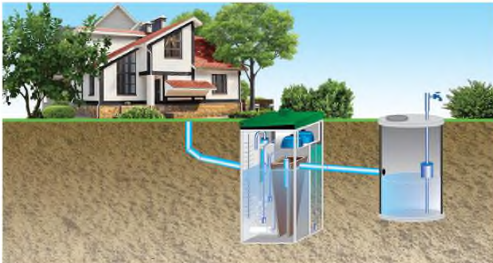
26-расм. Қайта фойдаланиш учун тўпланган резервуарга тозаланган сувни ўтказиш схемаси
